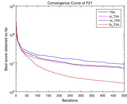
(d) f_{21} , Hybrid Function
