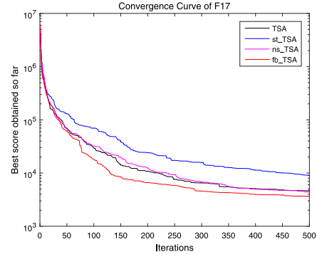
(d) f_{17} , hybrid function
