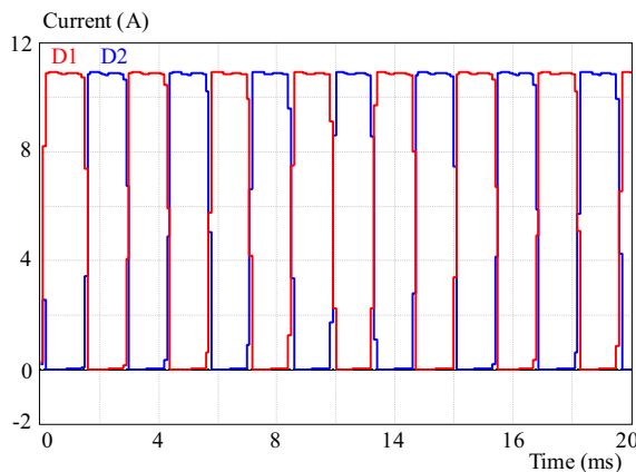
Fig. 8. Diode D1 and D2 current waveforms
