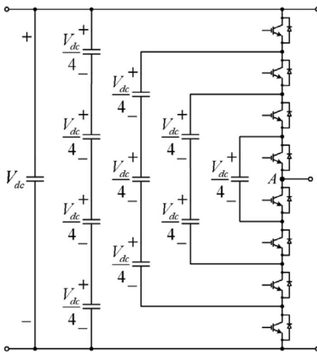
Fig. 13. Five-level FC VSC phase leg.
